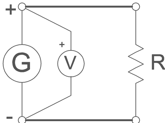
SCHEMA PER MISURA DI TENSIONE (V) IN UN SEMPLICE CIRCUITO
