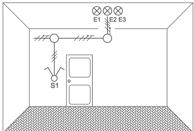
SCHEMA UNIFILARE
