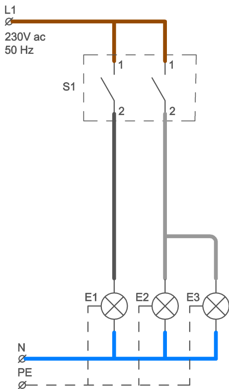
SCHEMA FUNZIONALE
